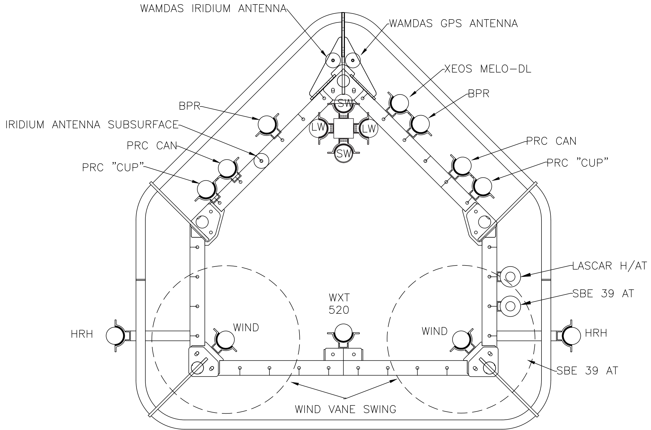
NTAS 16 TOWER TOP V2 10/18/16 BP
